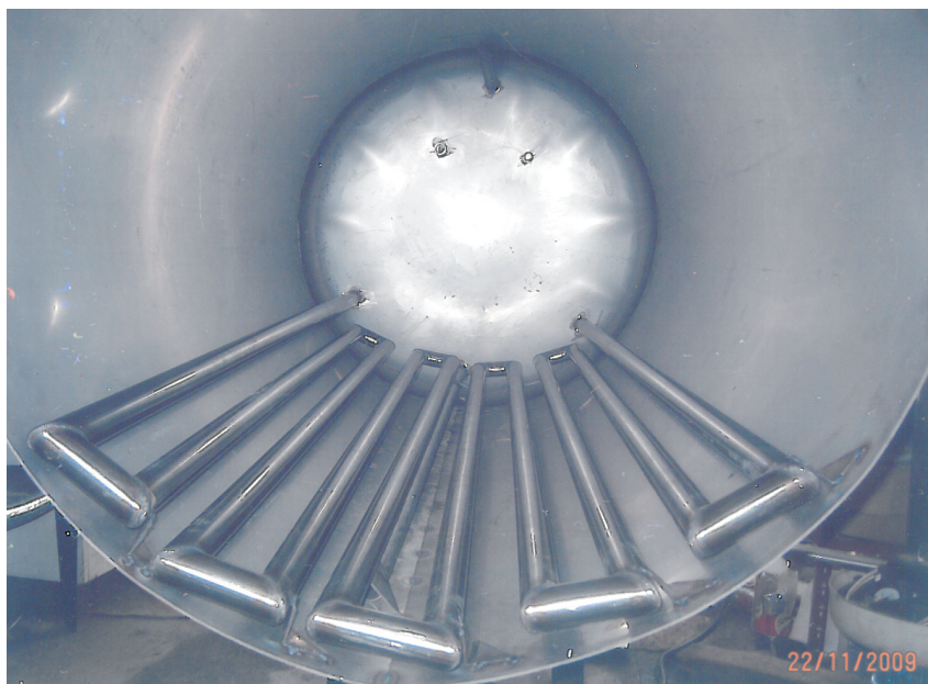
ЛИРА ЗА ХОРИЗОНТАЛЕН БОИЛЕР
